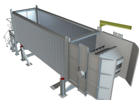
Trémie Doseuse sur Pesons
