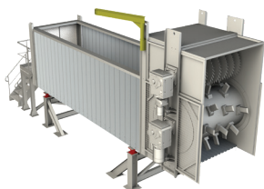
Trémie Ouvre-sacs sur Pesons
